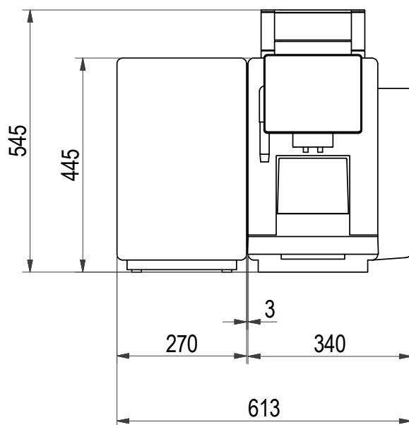
A300/SU05 mit Wassertank und Pulverbehälter
